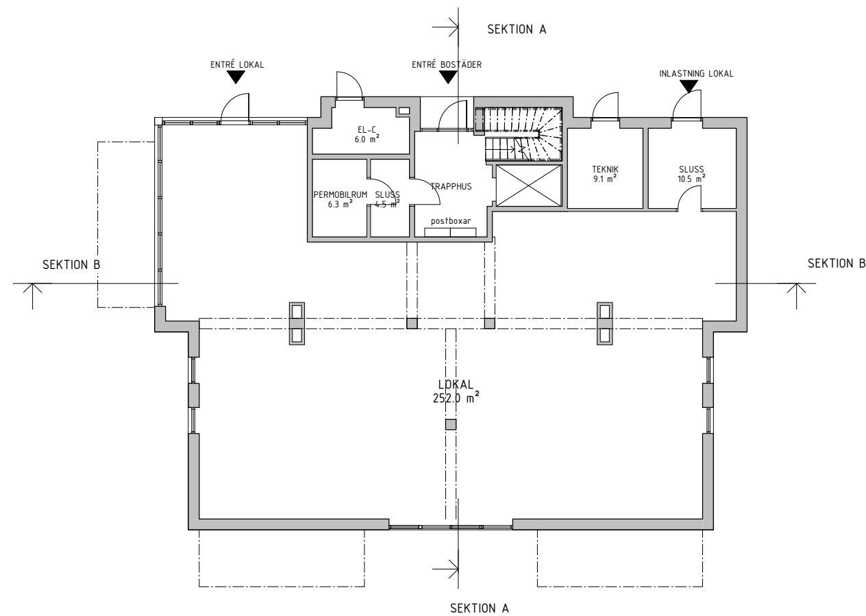
VÅNING 1
