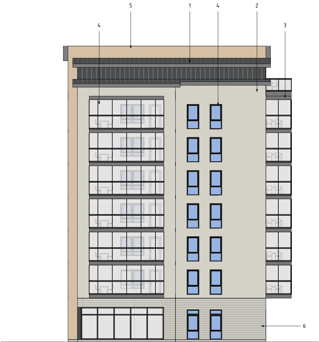
FASAD MOT VÄSTER
