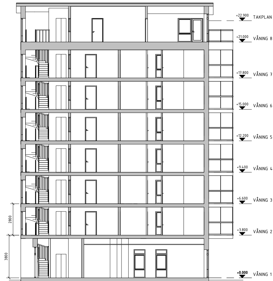
SEKTION A
