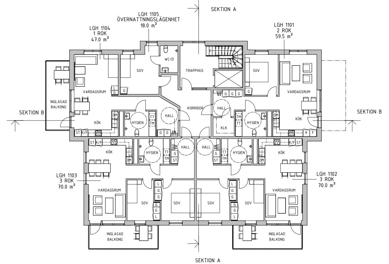
VÅNING 2
