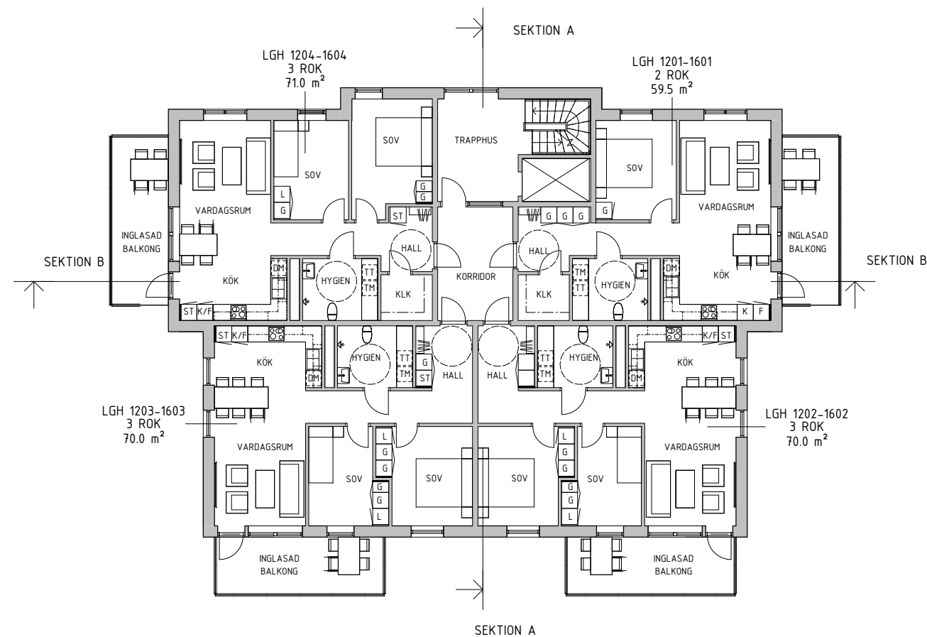
VÅNING 3
